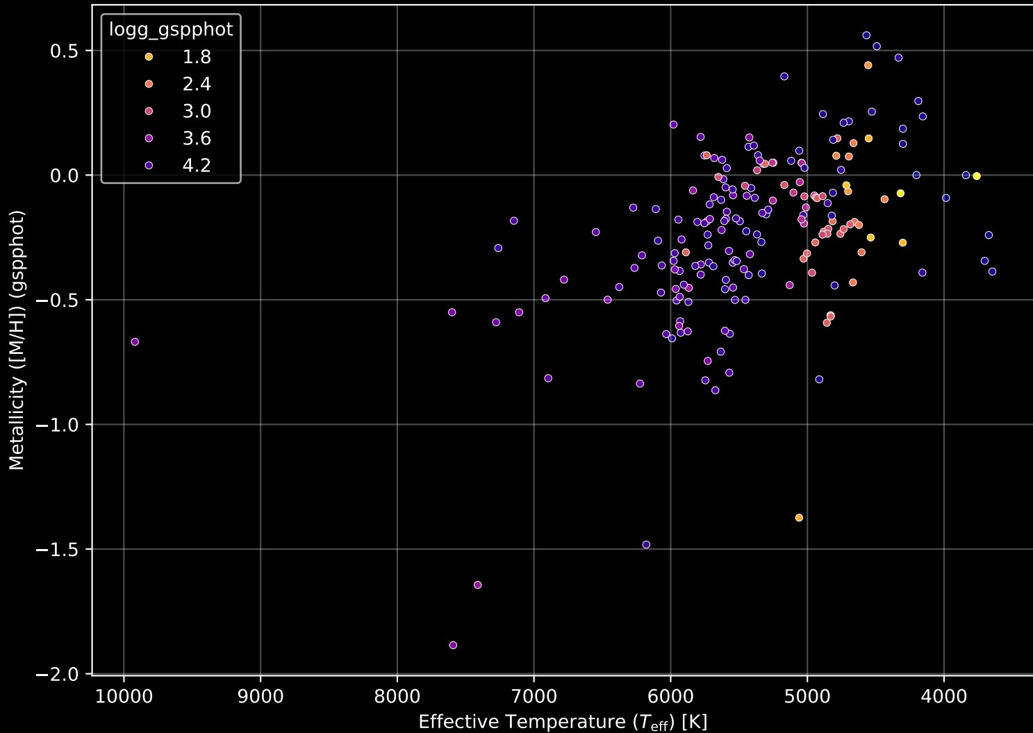
APOGEE DR17 Field: [164+32_MGA] Stellar Population Parameters (n= 194)
